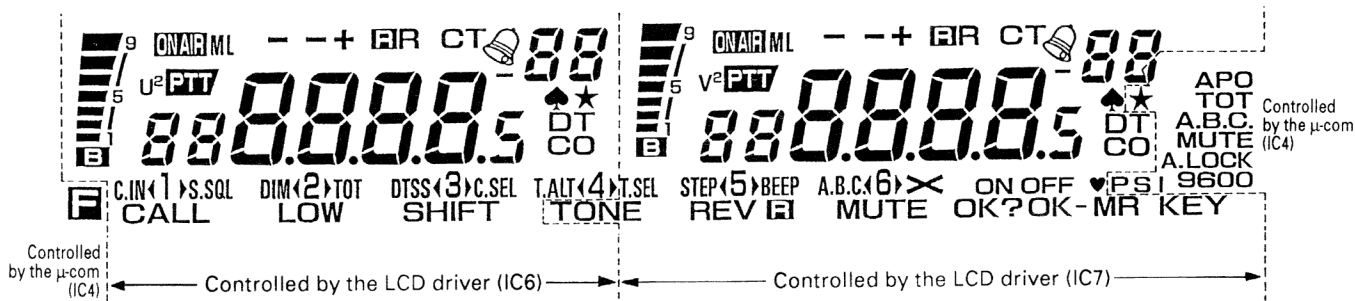
Fig. 18 Display LCD (Except M4 type)
